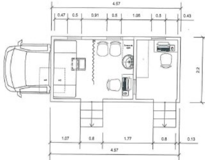
Distribución del furgón de carga seca
